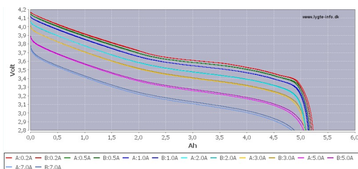
Charakterystyka rozładowania akumulatora XTAR 26650
