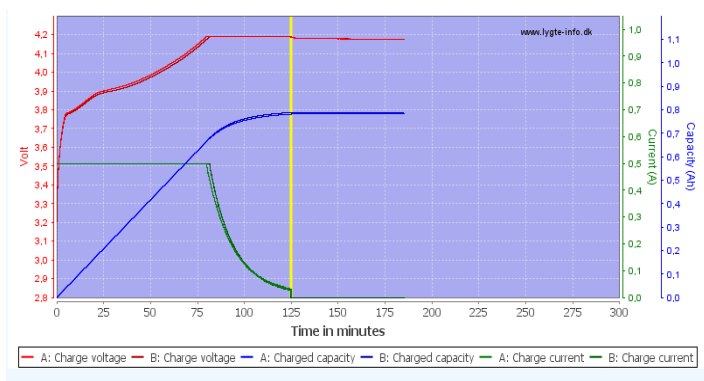
Charakterystyka ład. akumulatora : KP ICR14500-110PCM
