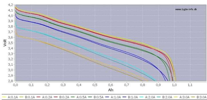
Charakterystyka rozład. akumulatora : KP ICR14500-110PCM
