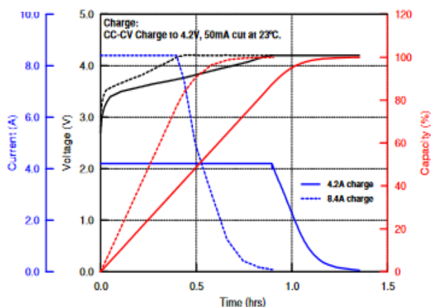
Charakterystyka ładowania akumulatora : MOLI INR21700-P42A 4200mAh
