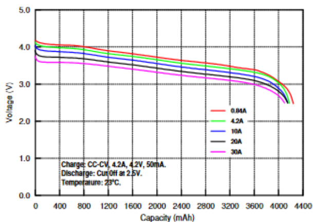
Charakterystyka rozładowania akumulatora : MOLI INR21700-P42A 4200mAh
